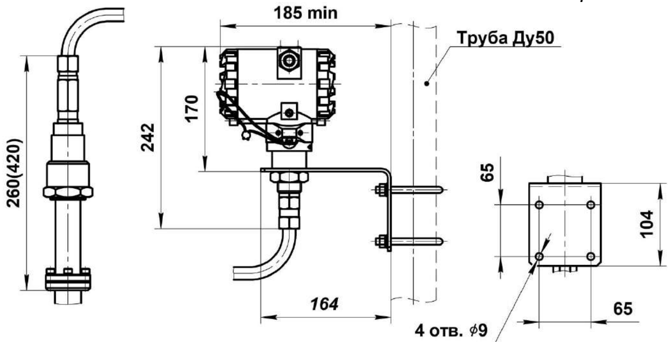
Рисунок В.13 – Размеры расходомеров дистанционного исполнения. Остальные размеры см. Рис.В.1 ...В.12
